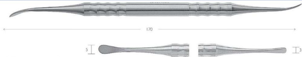
KN 27.721.02 MOLT FIG. 2
